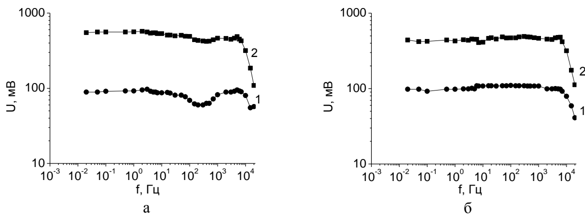
Частотные зависимости пирооткликов при нагреве (а) и охлаждении (б) для пленок с асимметричными (1) и симметричными (2) электродами
