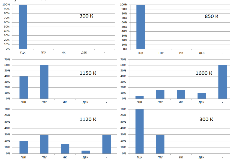
Изменение распределения локальной структуры в нанокластерах Au, содержащих 2000 атомов, в ходе процесса плавления-кристаллизации
