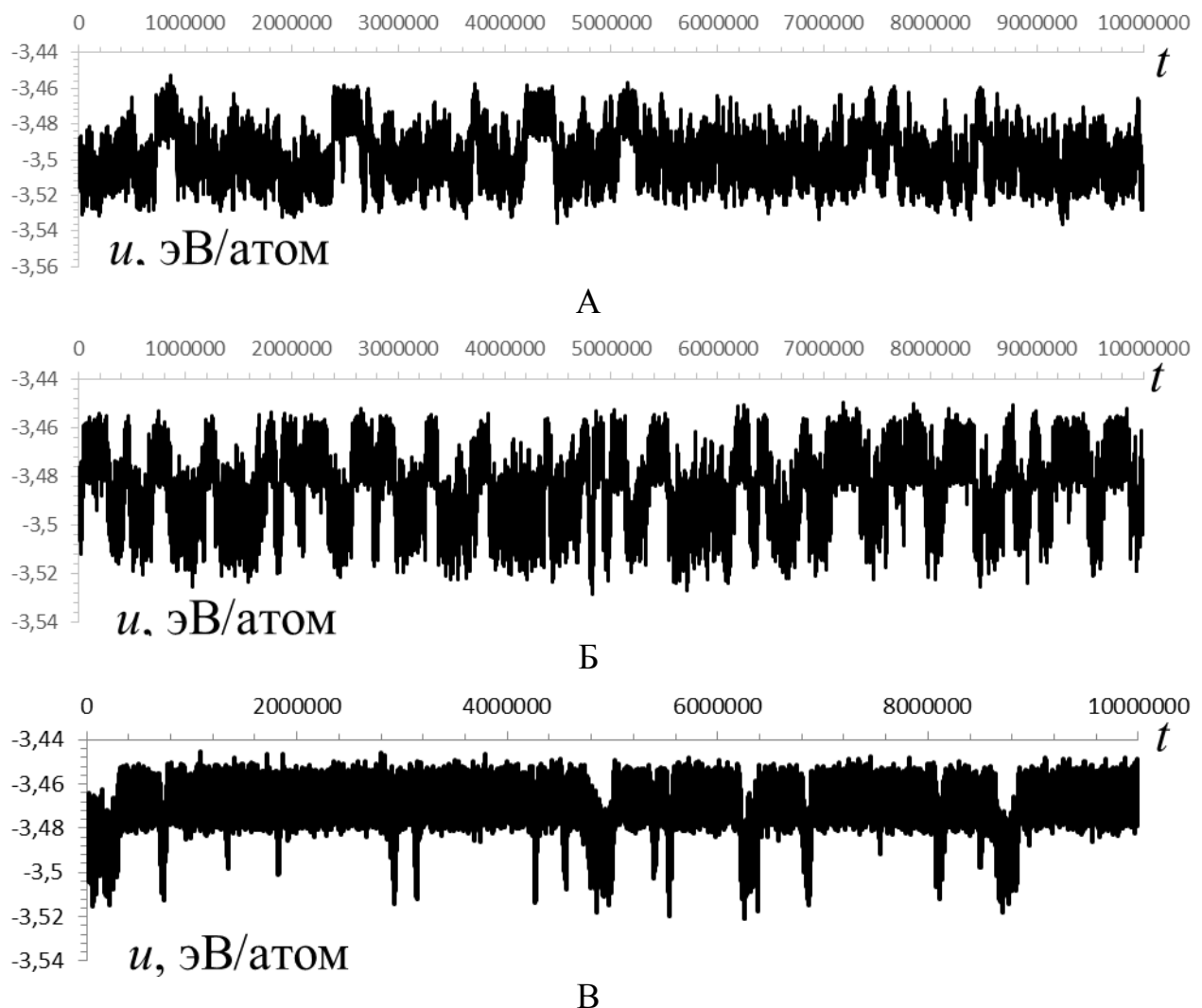
Рис. Изменение потенциальной части внутренней энергии u с увеличением шага для нанокластера золота содержащего N=1000 атомов при различных температурах: а) T=875\text{K} ; б) T=900\text{K} ; в) T=925\text{K} .
